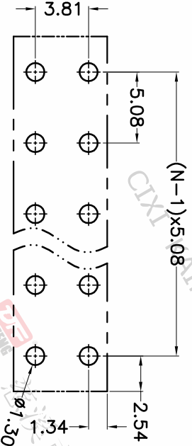
P.C.B.LAYOUT
